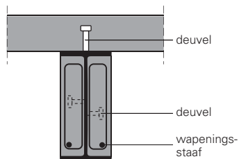
staal-beton ligger gedeeltelijk omstort
