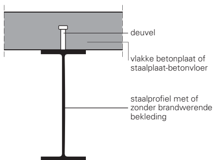
staal-beton ligger zonder betonomstorting
