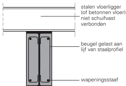
stalen ligger gedeeltelijk omstort
