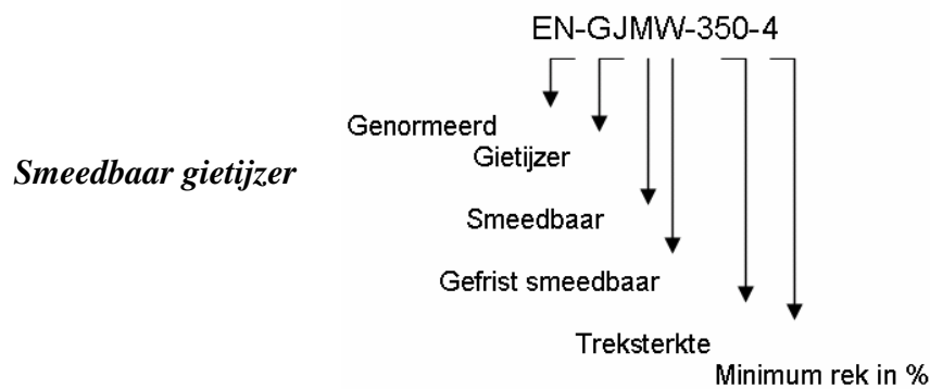
Figuur 6 symbolen smeedbaar gietijzer
