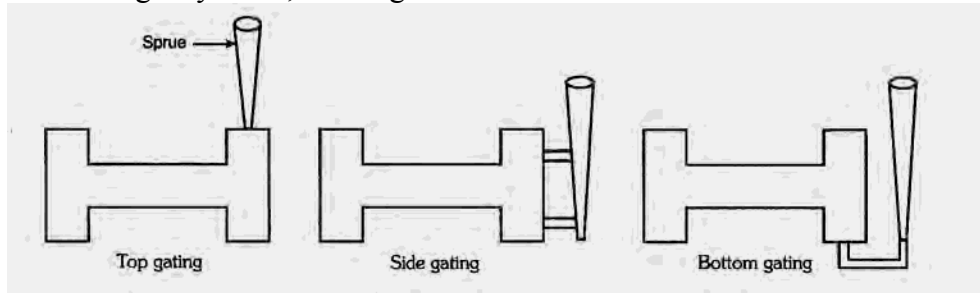
Figuur 32 orientatie gietsysteem, bron [7]
