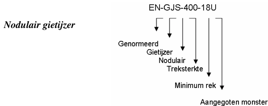
Figuur 7 symbolen nodulair gietijzer
