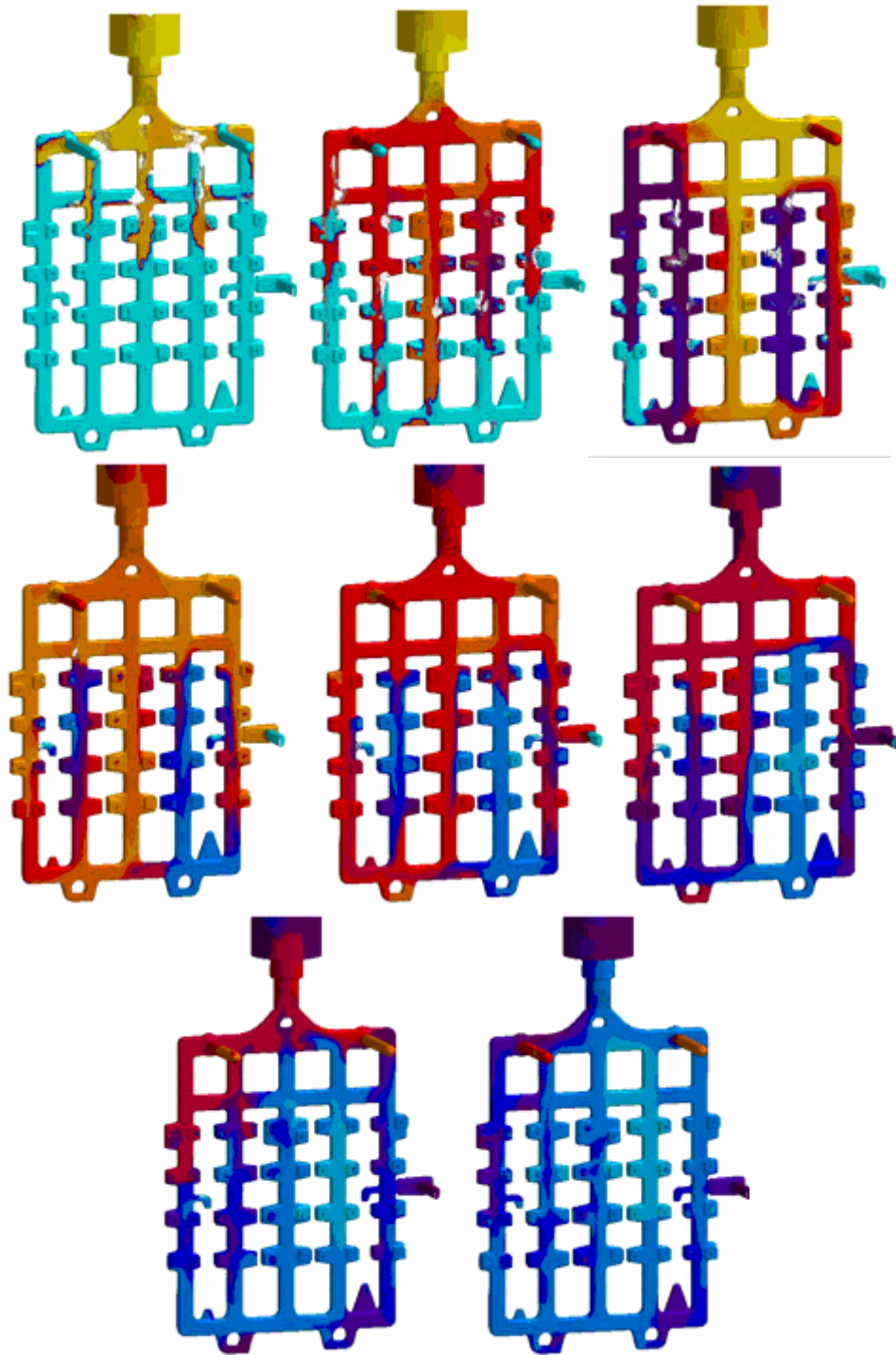
Figuur 64 Giet en stollingssimulatie
