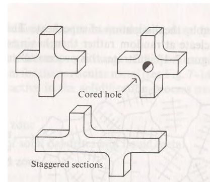
Figuur 41 voorkomen van hot spots, bron [8]
