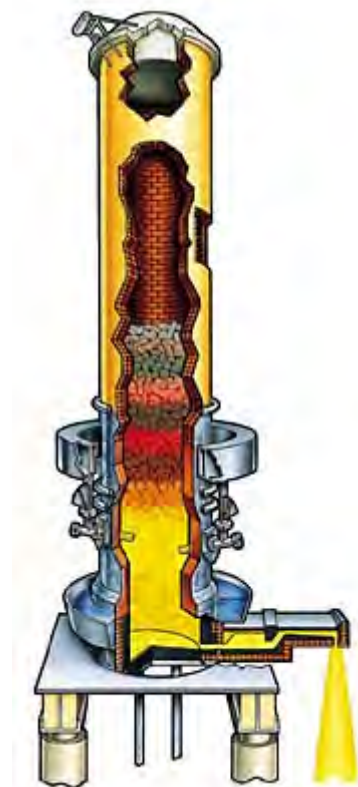
Figuur 18 Koepel oven, bron [74]
