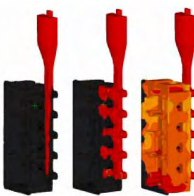
Figuur 66 drie fasen in gieten met temperatuur contouren, bron [52]
